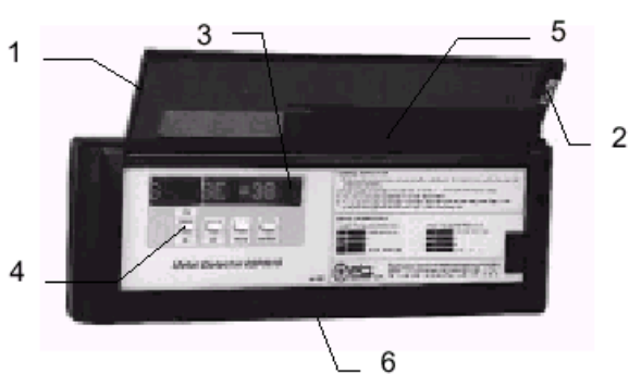
Рис. 1-2: Электронный блок управления модели 02PN10 в исполнении IP 20
