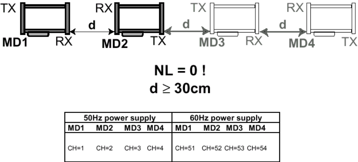
Рис. 2-3b Установка 3 или 4 металлодетекторов (d ≥ 30 см).
