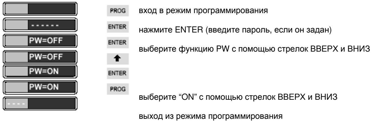
Рис. 3-7b Включение металлодетектора
