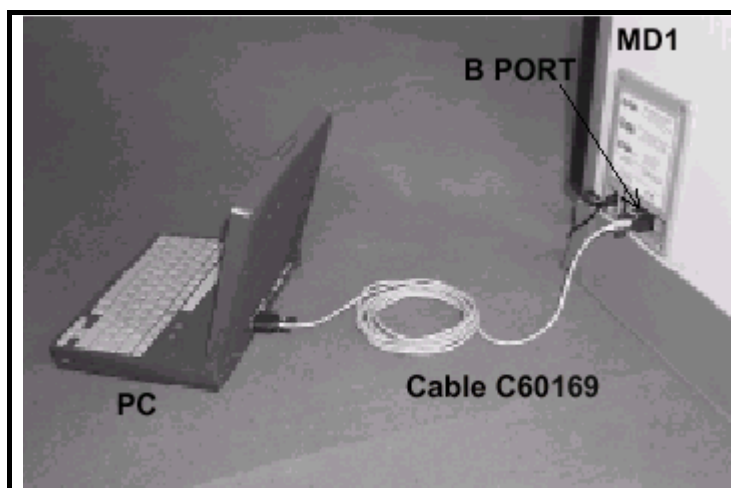
Рис. 4-4а Подключение к компьютеру
