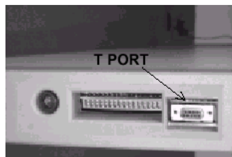
Рис. 4-5 Разъемы металлодетектора
