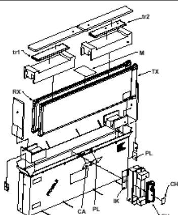
Рис. 2-5е Схема упаковки модели 02PN10
