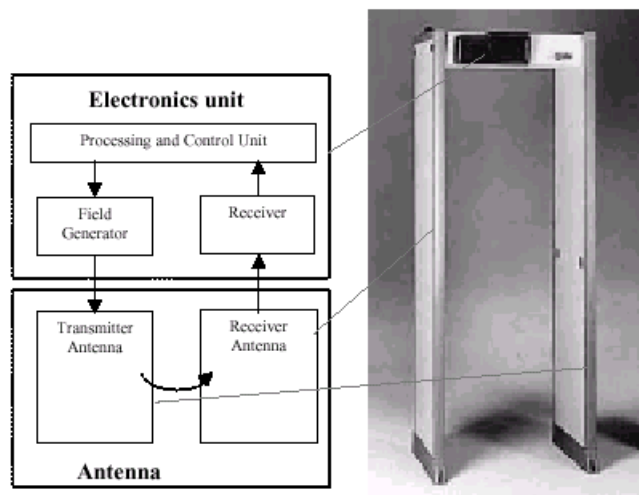
Рис. 1 Блок-схема металлодетектора
