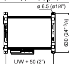
Рис. 2-5b Диаграмма отверстий для монтажа к полу (U+W=720/760/820 мм).
